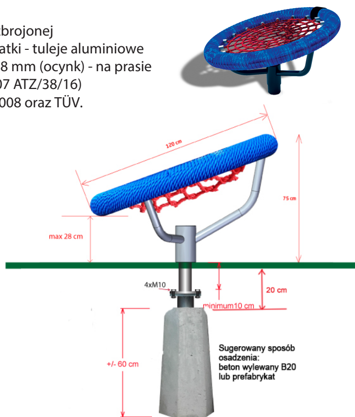
SCHEMAT MONTAŻU KARUZELI W GRUNCIE
