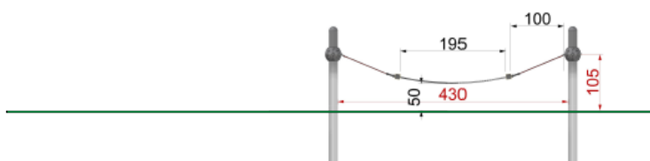
Wymiary hamaka lamelkowego
